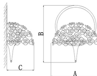
Model: CX-6106XL A : \varnothing 750 B : 900 C : 380 Source: E14*6 & LED 3W*2 Size : \varnothing 750 \times 900 \times 380 MM
