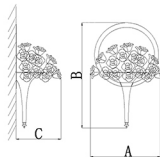
Model: CX-6106M A : \varnothing 400 B : 680 C : 250 Source: E14*4 & LED 3W*2 Size : \varnothing 400 \times 680 \times 250 MM
