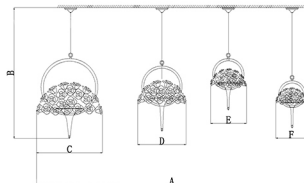
Model: CX-4866 (XL+L+M+S) A : 3000 B : 1450 C : \varnothing 750 D : \varnothing 550 E : \varnothing 400 F : \varnothing 350 Source: E14*30 & LED 3W*10 Size : 2400*800 MM
