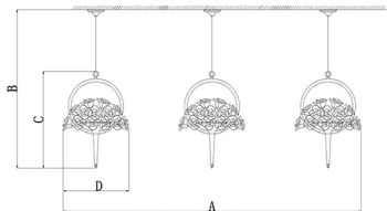
Model: CX-4866 (L+L+L) A : 2400 B : 800 C : 1200 D : \varnothing 550 Source: E14*27 & LED 3W*9 Size : 2400*800 MM
