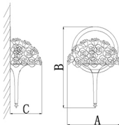
Model: CX-6106S A : \varnothing 350 B : 600 C : 200 Source: E14*3 & LED 3W*2 Size : \varnothing 350 \times 600 \times 200 MM
