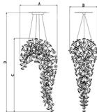
Model: CX-6914L A : 1000 B : 700 C : 2000 D : 2500 Source: E14 * 19 Size : 1000*700*2000 MM
