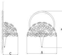
Model: CX-6106XXL A : \varnothing 1000 B : 1150 C : 400 Source: E14*7 & LED 3W*3 Size : \varnothing 1000 \times 1150 \times 400 MM
