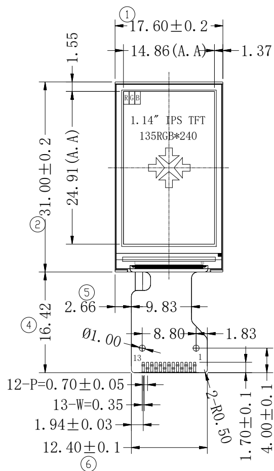
正视图
