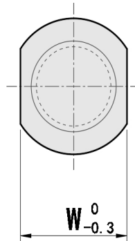
W < V, Y ≥ 17时的两平面宽度尺寸 Dimensions of Wrench Flats when W < V, Y ≥ 17
