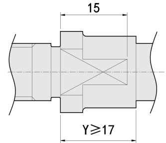
W < V, Y ≥ 17时的两平面宽度尺寸 Dimensions of Wrench Flats when W < V, Y ≥ 17
