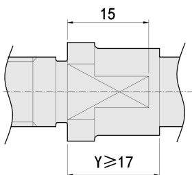
W < V, Y ≥ 17时的两平面宽度尺寸 Dimensions of Wrench Flats when W < V, Y ≥ 17
