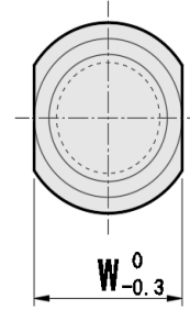
W < V, Y ≥ 17时的两平面宽度尺寸 Dimensions of Wrench Flats when W < V, Y ≥ 17
