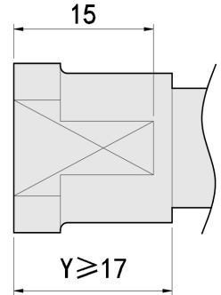
W < V, Y ≥ 17时的两平面宽度尺寸 Dimensions of Wrench Flats when W < V, Y ≥ 17
