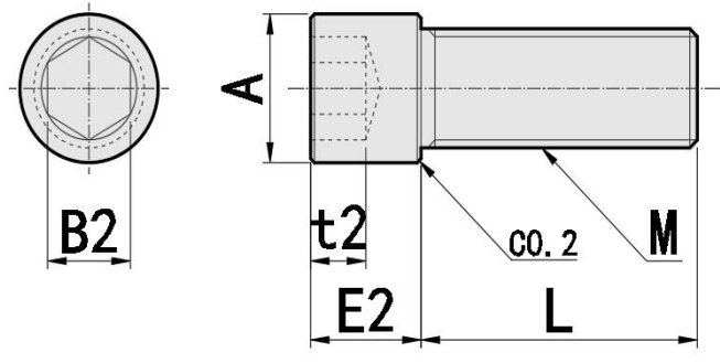
小径头螺栓/Small Head Cap Screws ZSBB / ZSBBSS
