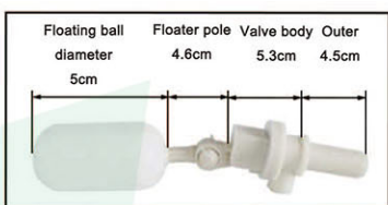
YH-AF118A Floating ball
