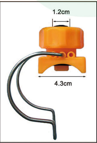
YH-CT149-1 Base Φ50
