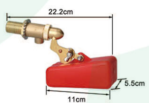
YH-AF119 Floating ball
