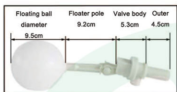
YH-AF118B Floating ball
