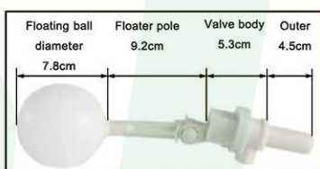
YH-AF118C Floating ball
