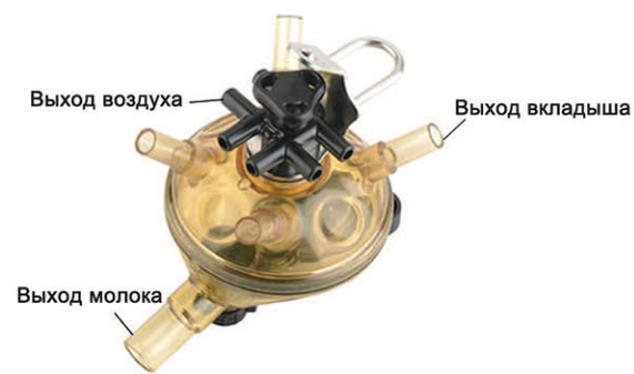
IPC300 Молочный коллектор УН-МЕ361ВАА
