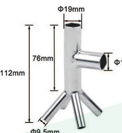
YH-ME231 S.S. 分配器
