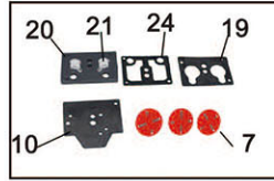
YH-ME071S4 YH-ME071A/ME071B专用
