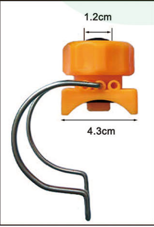
YH-CT149-1 管径 Φ50
