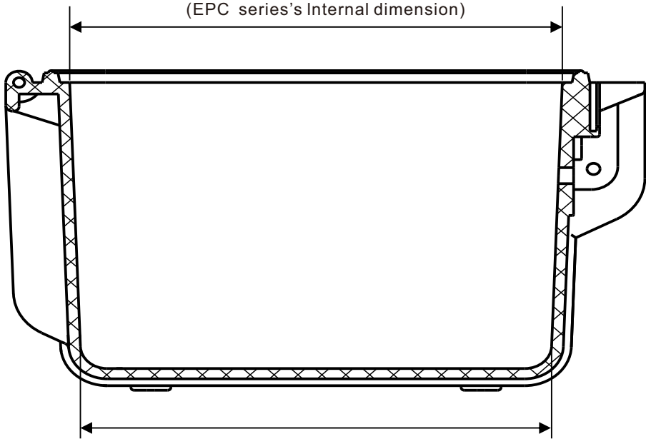
RPC系列内部尺寸标注位置 (RPC series's Internal dimension)
