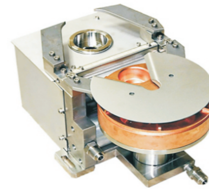
> 电子束蒸发源 < Electron beam evaporation source
