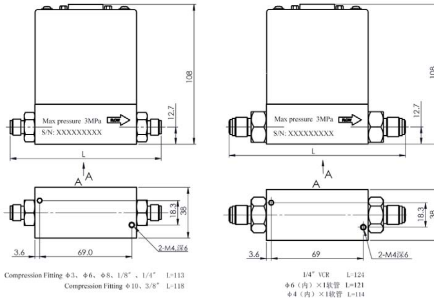
图 4. D07-19B、D07-19BM 型 MFC 和 MFM 外形尺寸
