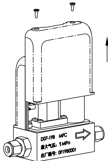
图 13. D07-19B、D07-19BM 型外罩安装图
