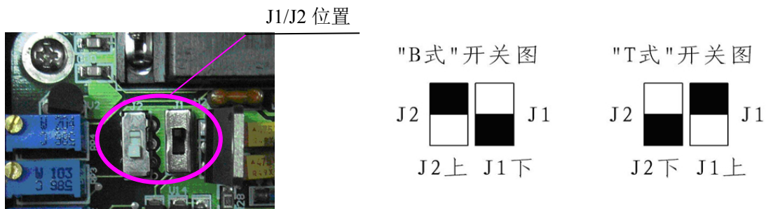
图 8. D07-19B 型 MFC 插座引线开关位置图
