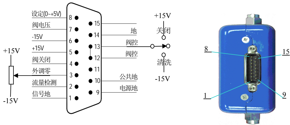
图 7. D07-19B 型 MFC 的“B 式”接线图
