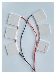
TEM Array 致冷片多片串并联
