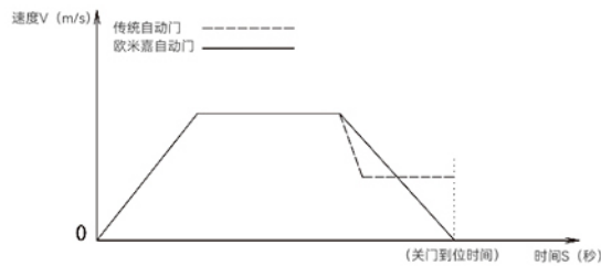
运行曲线示意图
