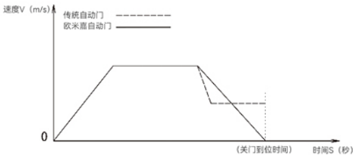
运行曲线示意图
