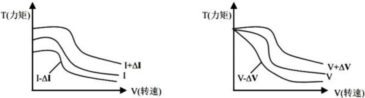
矩频特性图
