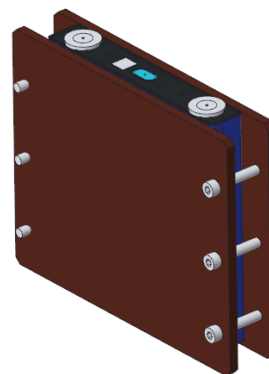
Fig. 4 Diagram of cell with clamp 图 4 电池上夹具图
