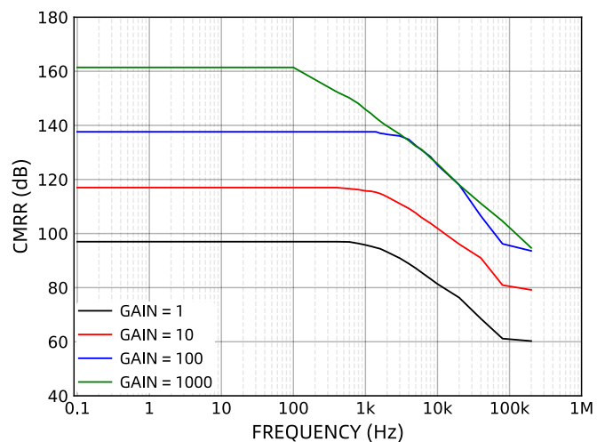
图 8 CMRR ( G = 1 \sim 1000 )
