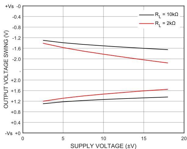
图 10 输入电压摆幅随电源电压的变化 ( G = 1 )
