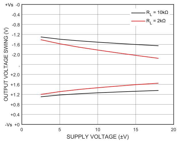
图 10 输出电压摆幅随电源电压的变化 ( G = 1 )
