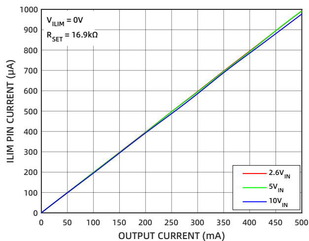
图 12 ILIM 管脚电流随输出电流的变化
