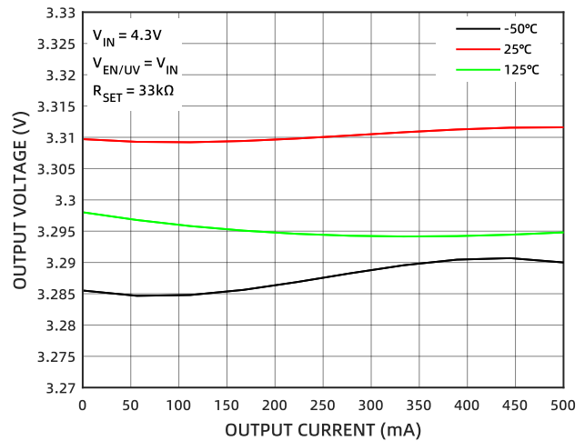
图 6 负载调整率
