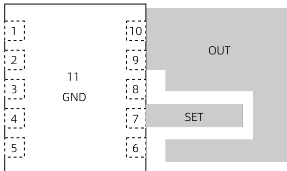
图 12 保护环布局
