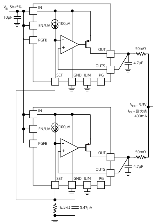
图 14 芯片并联
