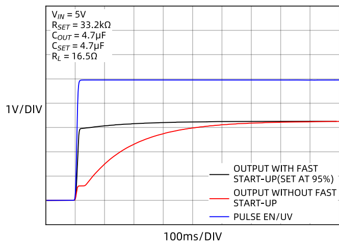
图 7 启动时间
