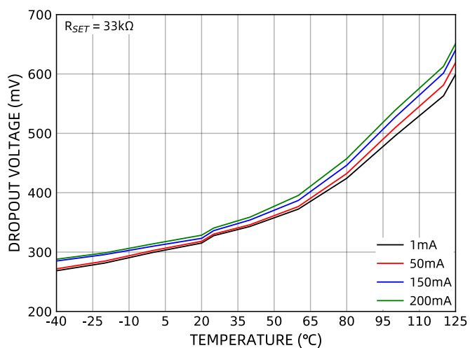
图 10 压差随温度的变化
