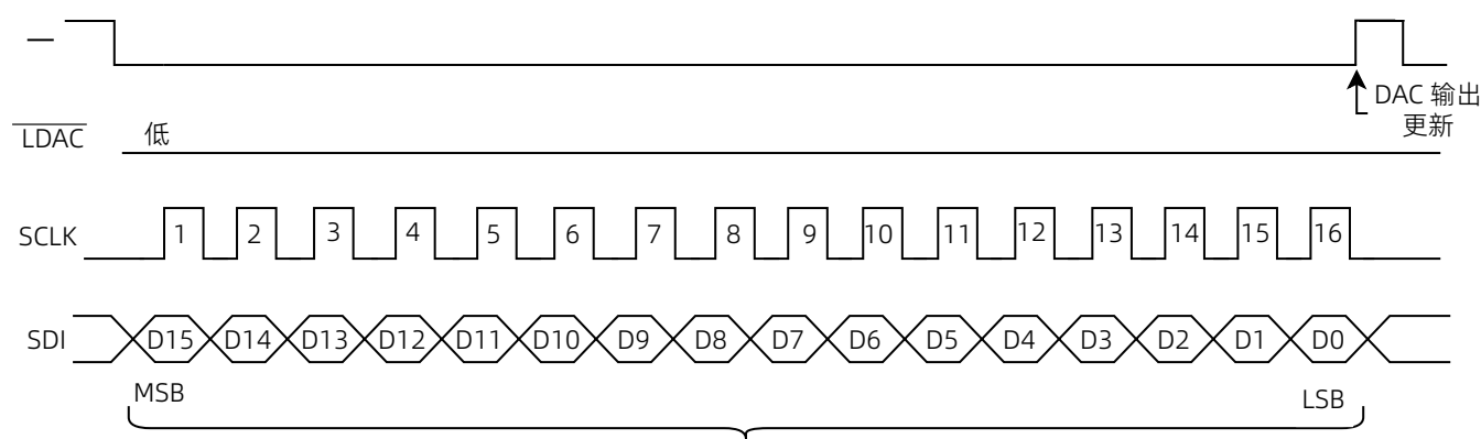
图 19 时序图
