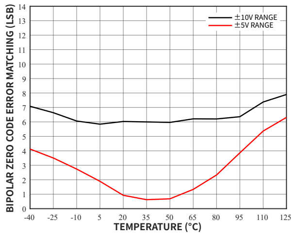
图 23 双极性 0 码误差匹配的温度特性
