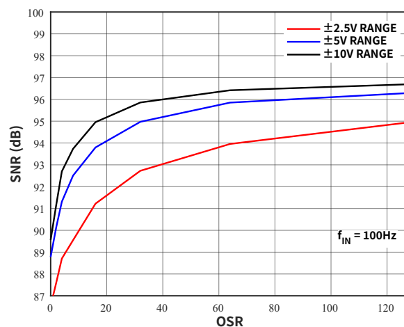
图 37 SNR 与 OSR 的关系图
