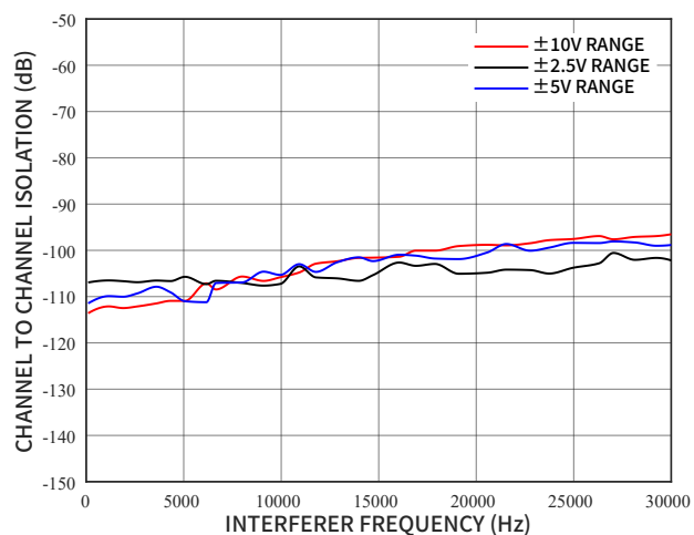
图 27 通道隔离度
