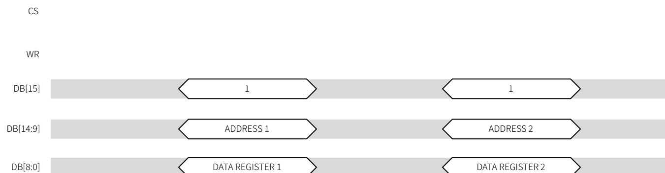
图 49 并行接口寄存器写操作
