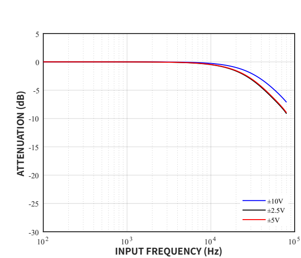
图 34 模拟抗混叠滤波器频率响应
