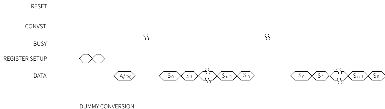
图 44 突发序列器软件模式
