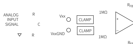
图 33 模拟输入电阻匹配
