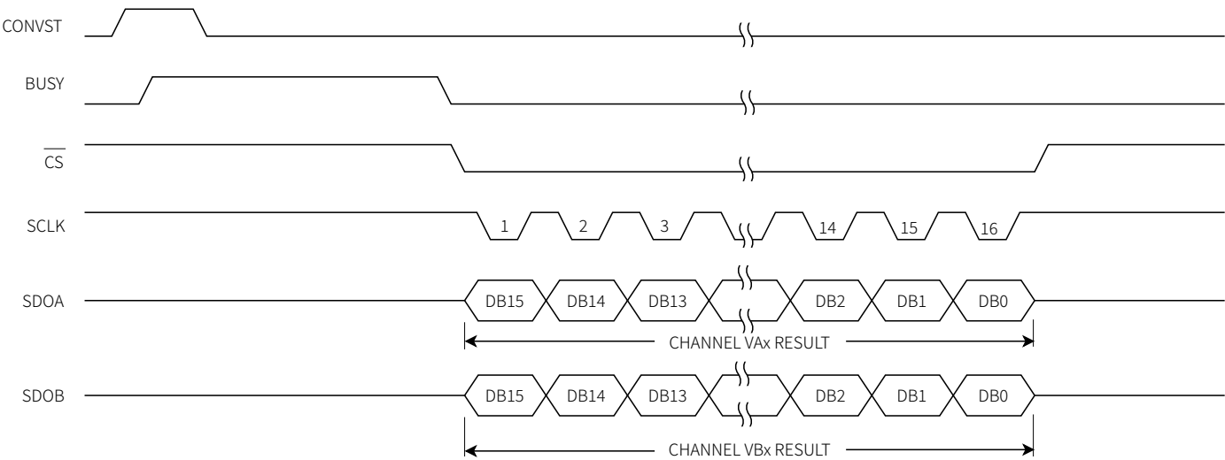
图 51 2 线串口模式转换结果读取
