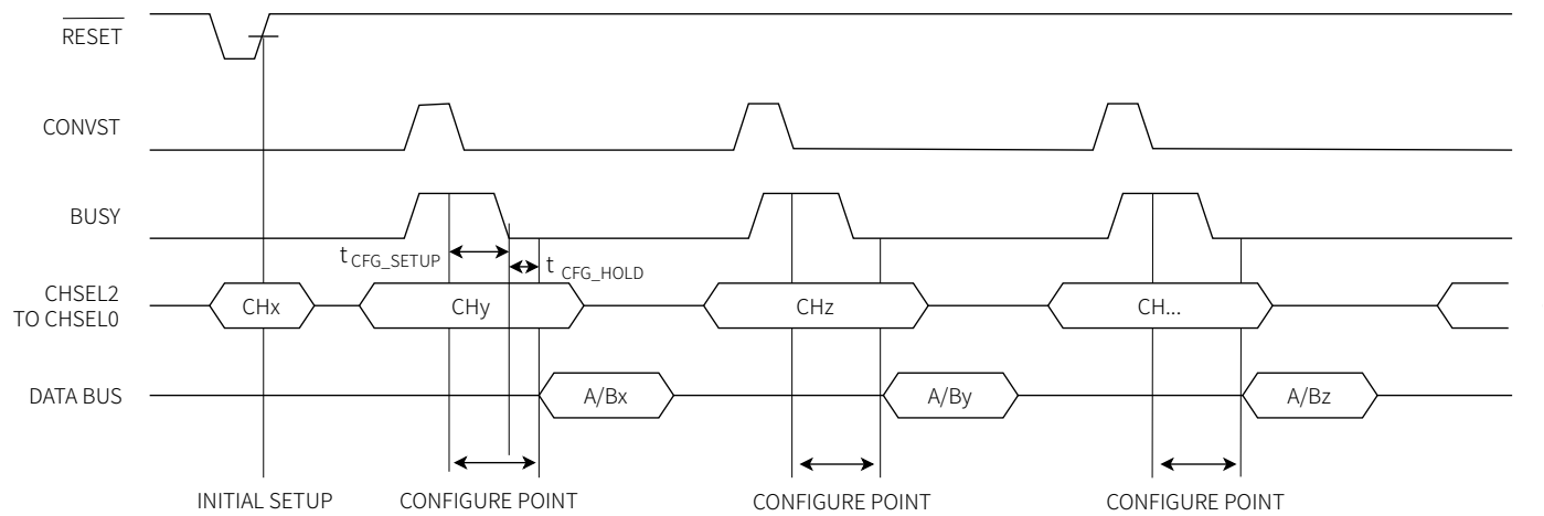
图 38 硬件模式通道转换设置图
