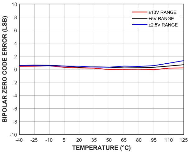
图 22 双极性 0 码误差的温度特性
