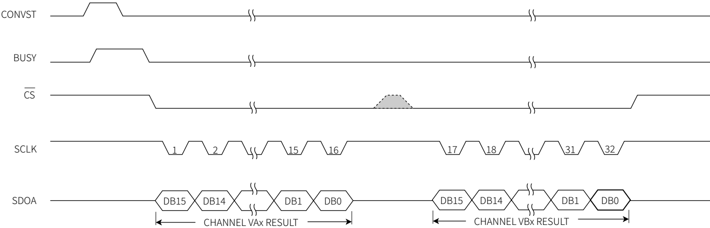
图 52 1 线串口模式转换结果读取
