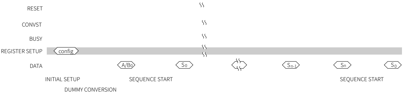
图 42 序列器软件模式
