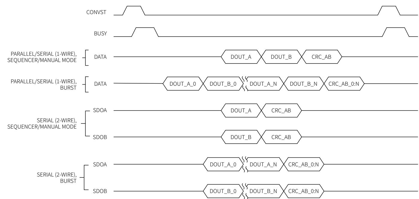
图 47 所有模式的 CRC 回读
