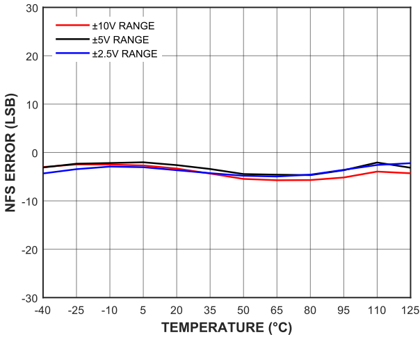
图 24 NFS 误差的温度特性
