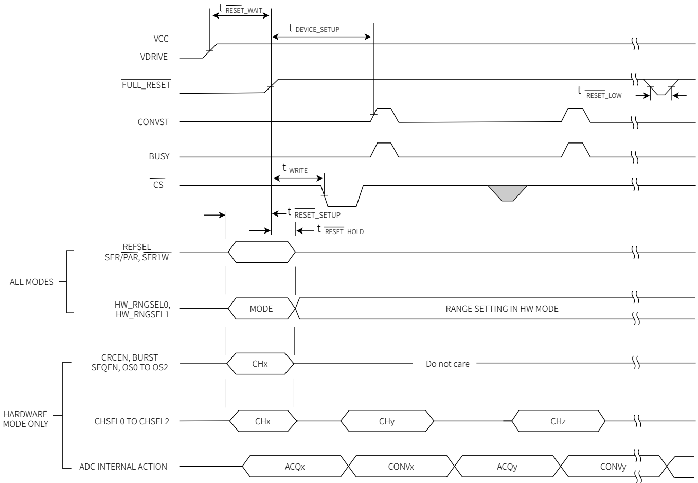
图 3 复位时序图
