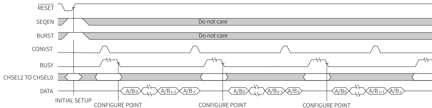
图 43 突发序列器硬件模式
