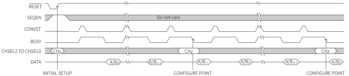
图 41 序列器硬件模式
