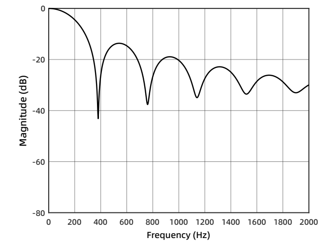
图 48 滤波器响应 (DR = 333SPS)
