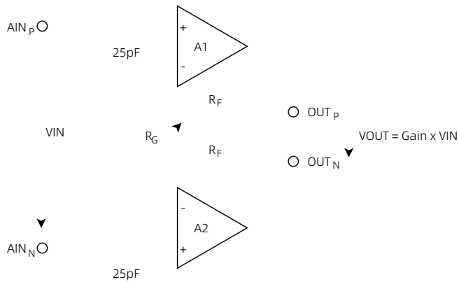
图 52 简化的 PGA 示意图
