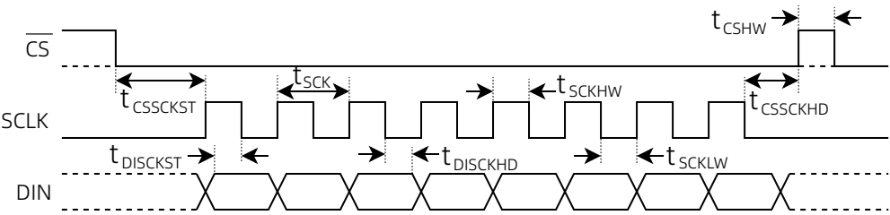
图 1 串行接口时序要求
