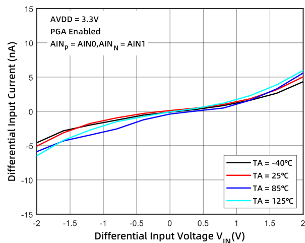
图 18 差分输入电流随差分输入电压的变化
