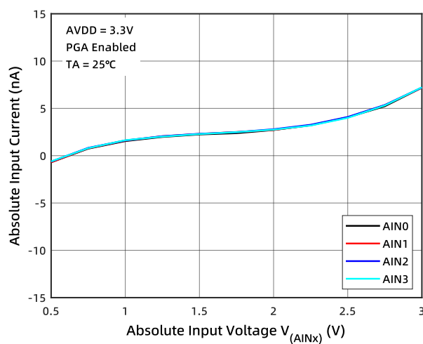
图 14 绝对输入电流随绝对输入电压的变化
