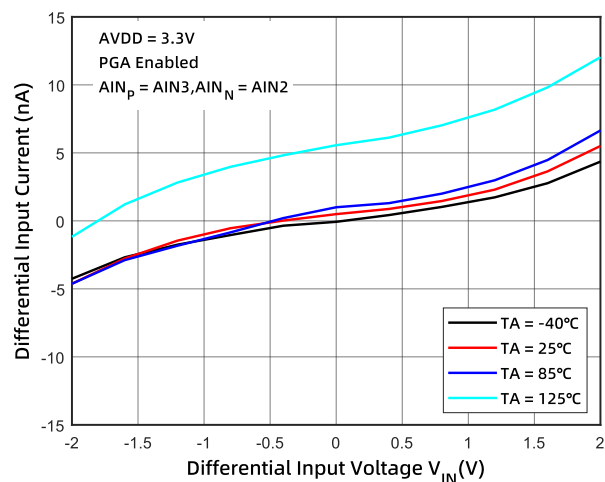
图 17 差分输入电流随差分输入电压的变化
