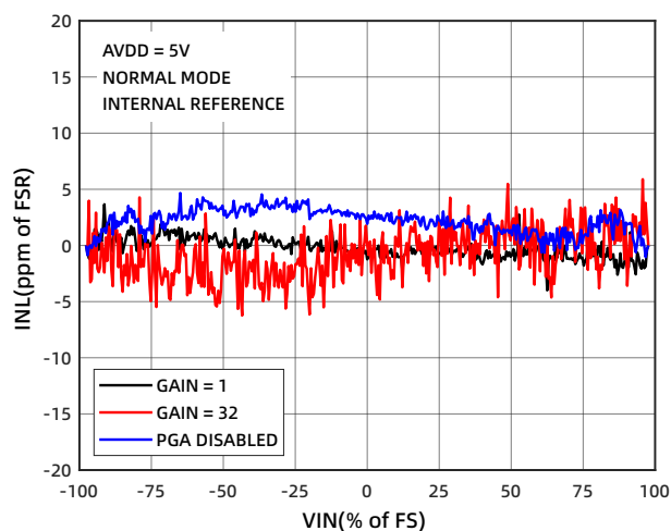
图 10 INL 随差分输入信号的变化
