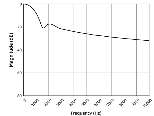
图 50 滤波器响应 (DR = 1kSPS)
