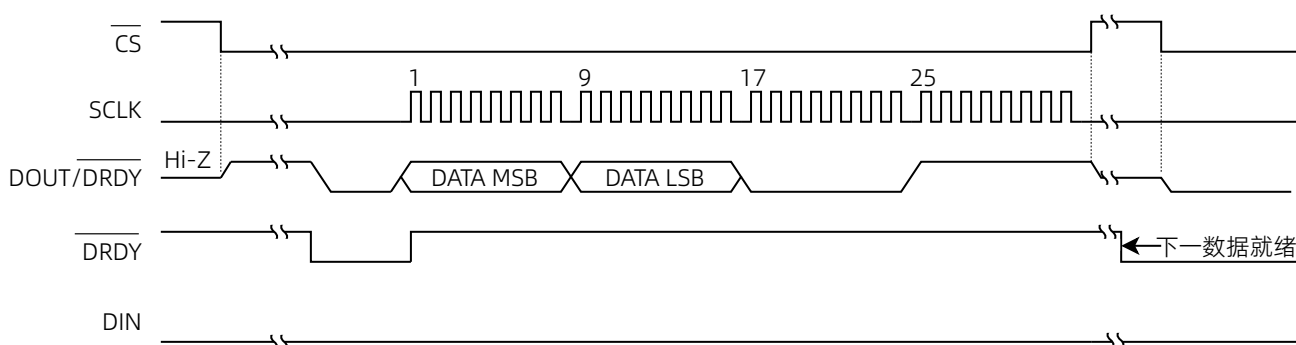
图 66 在读取转换结果后将 DOUT/DRDY 驱动为高电平的示例
