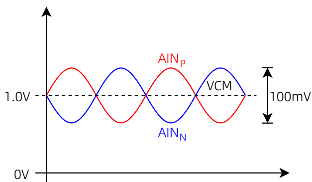
图 57 全差分输入信号
