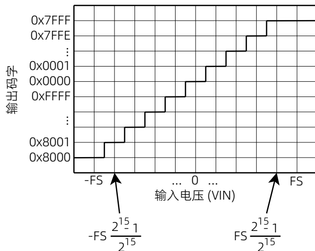
图 59 码字转换图
