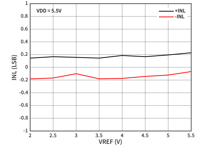
图 4 INL 随 VREF 的变化
