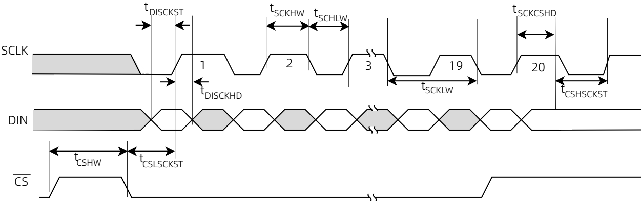
图 1 SPI 时序图
