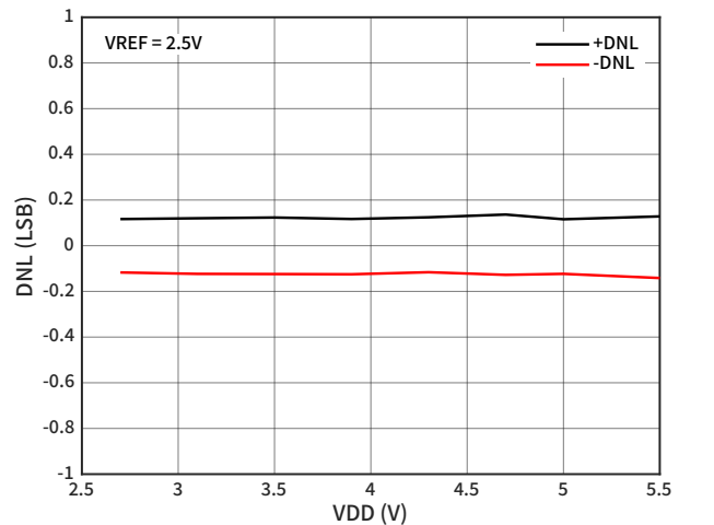
图 7 DNL 随 VDD 的变化
