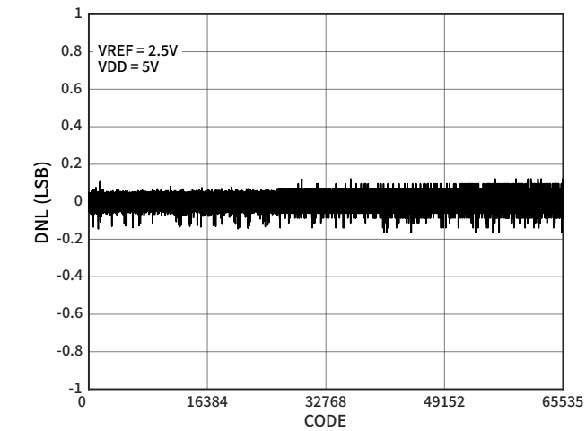
图 6 DNL
