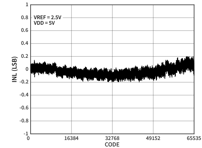
图 2 INL
