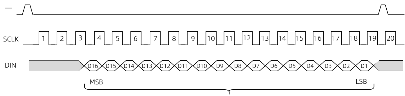
图 23 时序图
