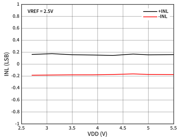
图 3 INL 随 VDD 的变化
