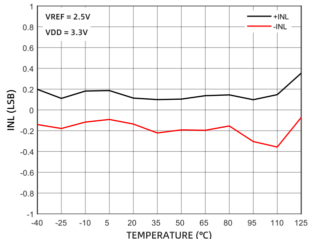
图 5 INL 的温度特性
