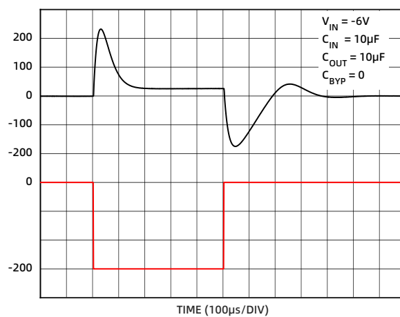
图 12 瞬态响应( C_{BYP} = 0nF , CM6511-5)
