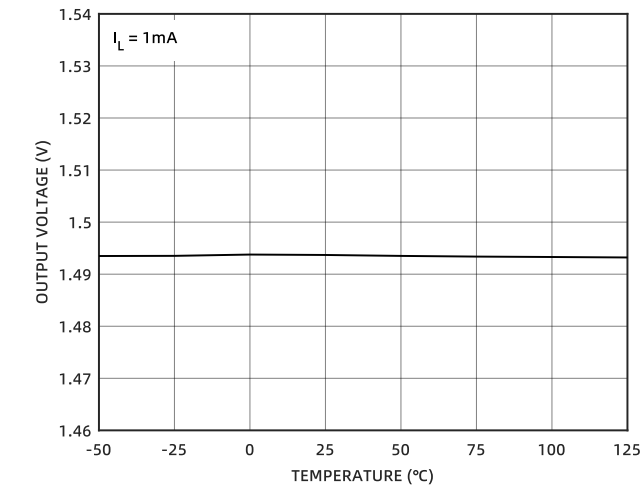
图 3 输出电压的温度特性 (CM6140)
