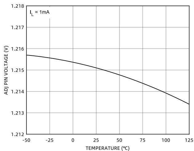
图 7 ADJ 管脚电压的温度特性 (CM6149)
