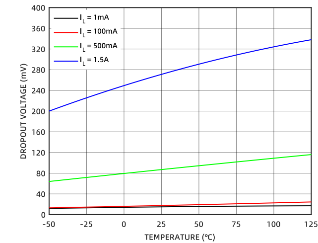
图 1 压差电压的温度特性
