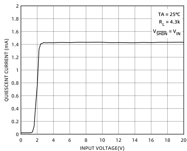
图 8 静态电流随输入电压的变化 (1.21V)
