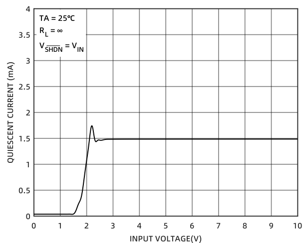
图 10 静态电流随输入电压的变化 (CM6141)
