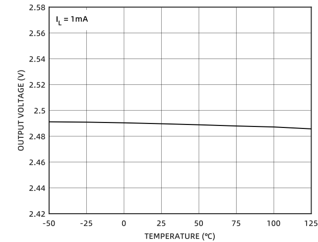
图 5 输出电压的温度特性 (CM6142)
