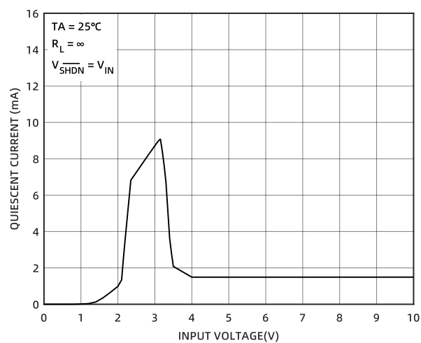
图 12 静态电流随输入电压的变化 (CM6143)
