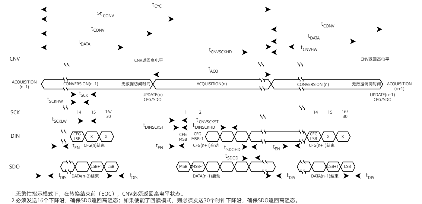
图 3 无繁忙指示器的串行接口时序
