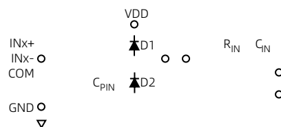
图 21 等效模拟输入电路
