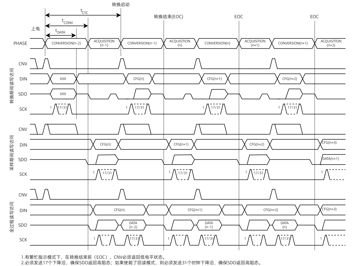
图 2 有繁忙指示器的通用接口时序
