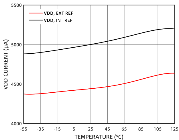
图 17 工作电流的温度特性
