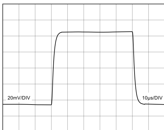
图 19 小信号响应 ( G = 100 , R_L = 2K\Omega , C_L = 100pF )
