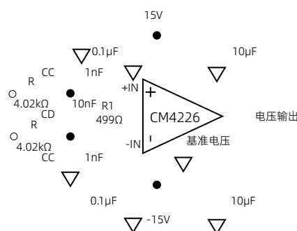
图 23 RFI 抑制
