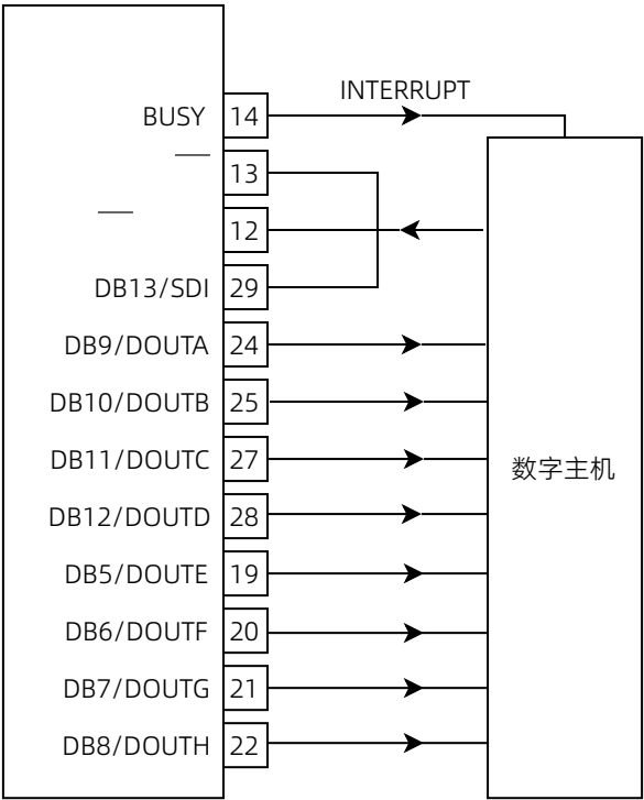
图 67 接口图-串行接口 8 条 DOUTx 线路
