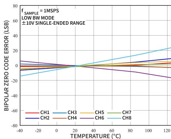
图 23 0 码误差的温度特性, \pm 10\text{V} 单端输入
