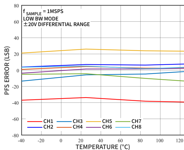
图 21 PFS 误差的温度特性, \pm 20\text{V} 差分输入
