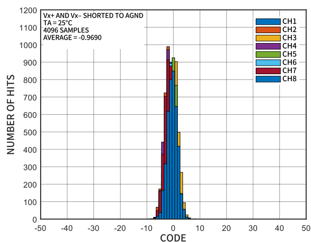
图 25 零输入直方图, \pm 10\text{V} 单端输入
