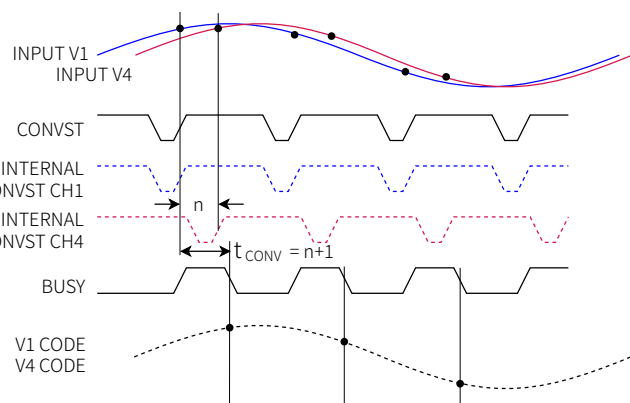
图 52 系统相位检测功能
