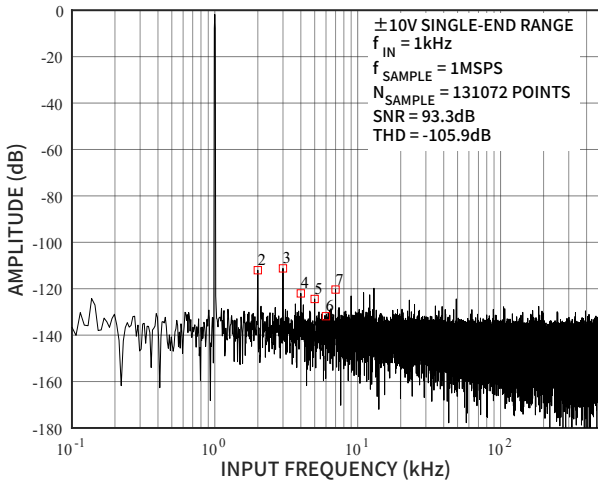
图 10 FFT, \pm 10\text{V} 单端输入, 低带宽模式
