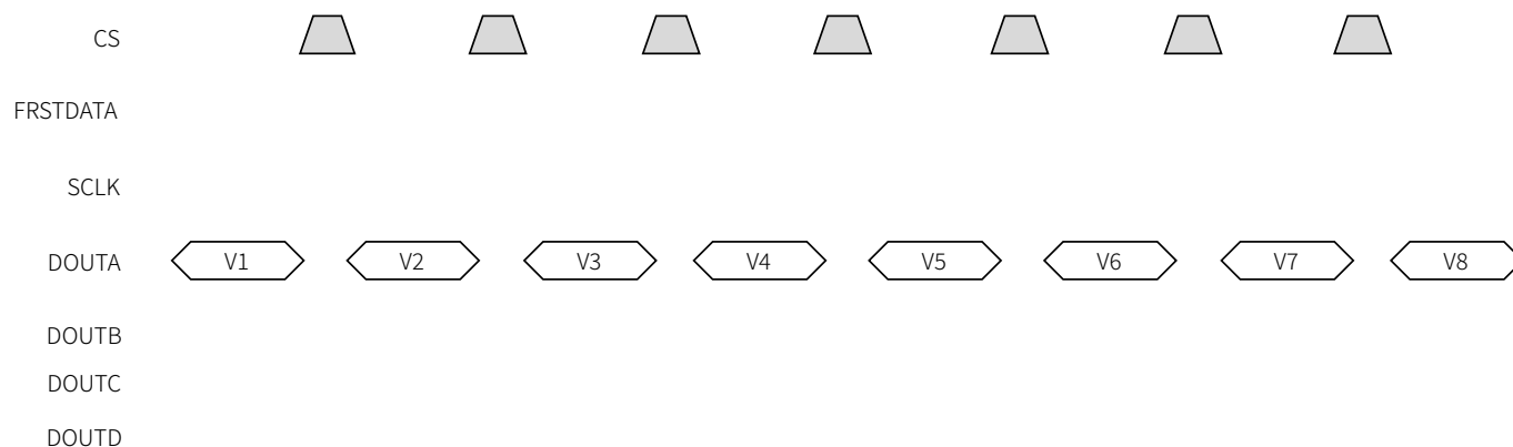
图 71 ADC 1 线读模式
