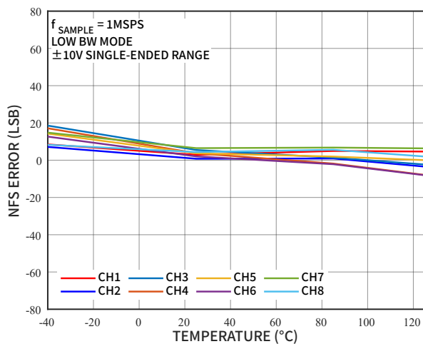
图 18 NFS 误差的温度特性, \pm 10V 单端输入
