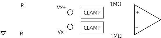
图 40 模拟输入端上的输入电阻匹配
