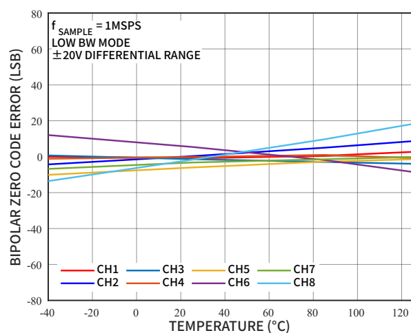
图 22 0 码误差的温度特性, \pm 20\text{V} 差分输入
