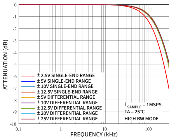
图 43 抗混叠滤波器幅频特性，高带宽模式
