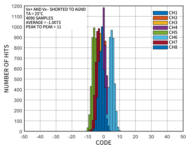
图 24 零输入直方图, \pm 20\text{V} 差分输入
