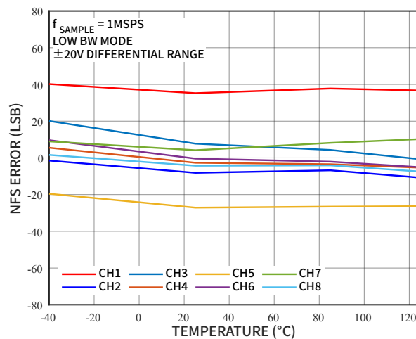
图 19 NFS 误差的温度特性, \pm 20V 差分输入
