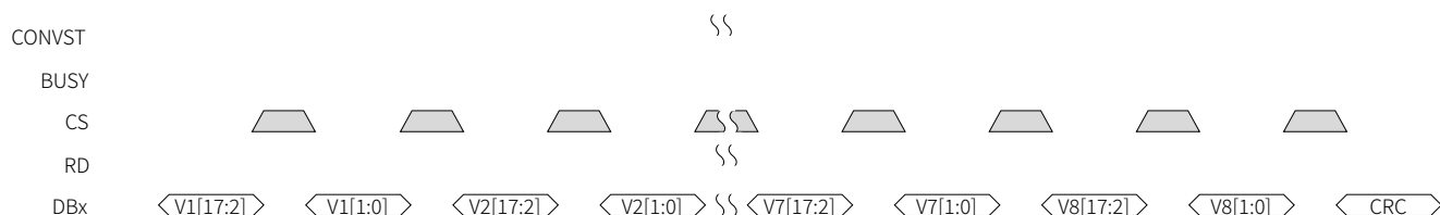
图 65 使能 CRC 后的 ADC 模式
