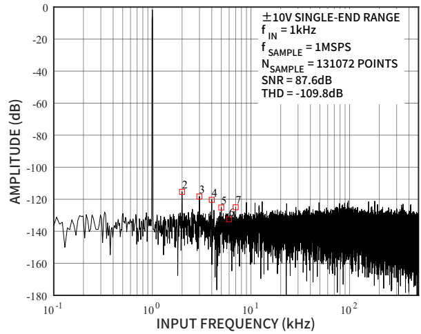
图 11 FFT, \pm 10\text{V} 单端输入, 高带宽模式
