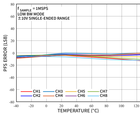
图 20 PFS 误差的温度特性, \pm 10\text{V} 单端输入
