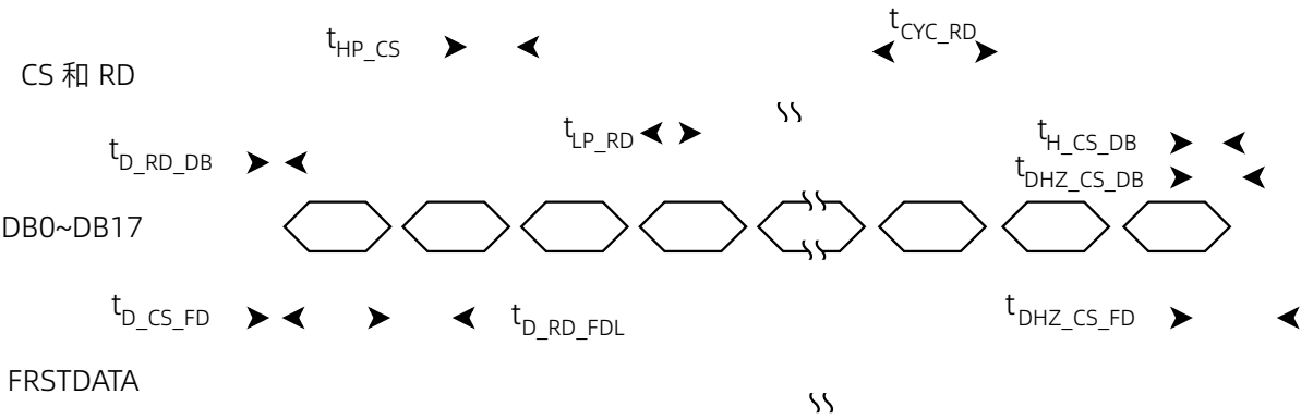
图 4 并行模式读取，相连的 \overline{CS} 和 \overline{RD} 脉冲
