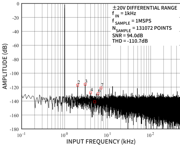
图 8 FFT, \pm 20\text{V} 差分输入, 低带宽模式
