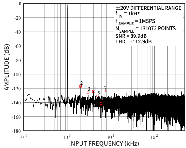
图 9 FFT, \pm 20\text{V} 差分输入, 高带宽模式
