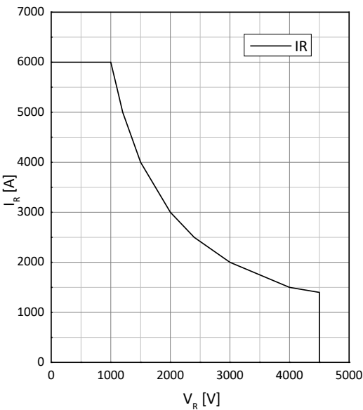
二极管安全工作区 safe operating area diode (RROA)
