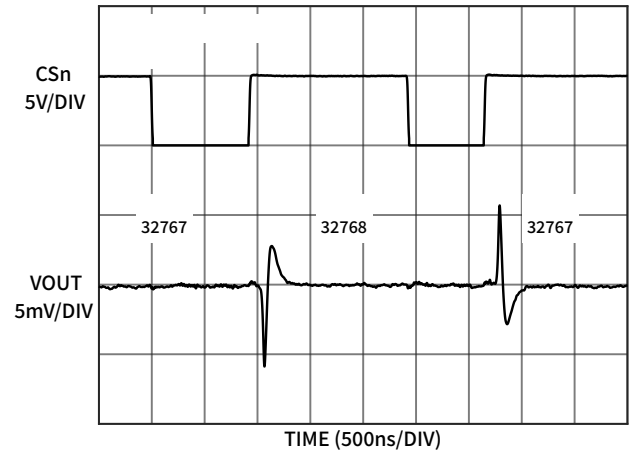
图 20 主进位翻转毛刺脉冲
