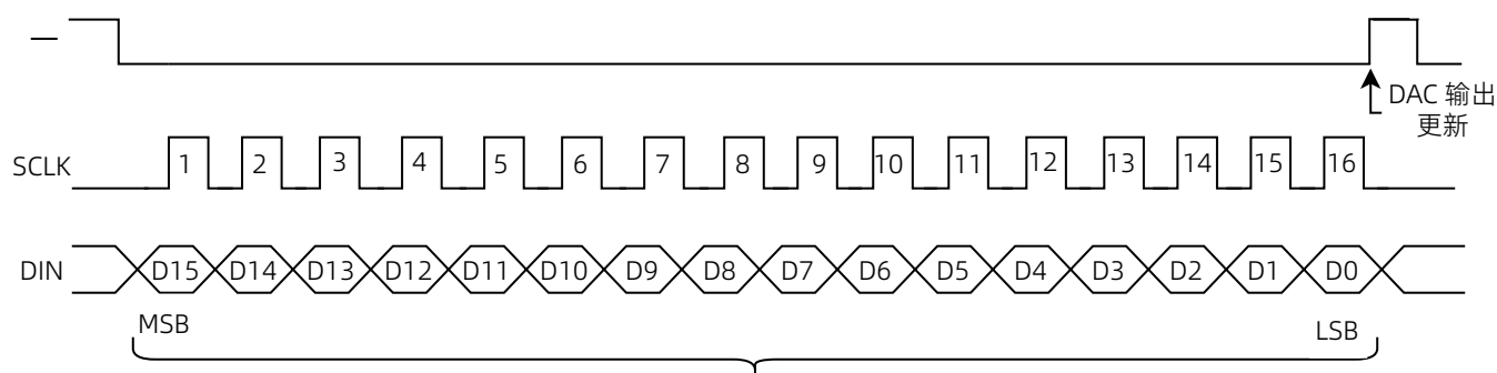
图 25 时序图
