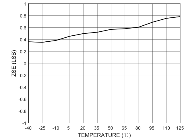
图 22 零码失调误差的温度特性
