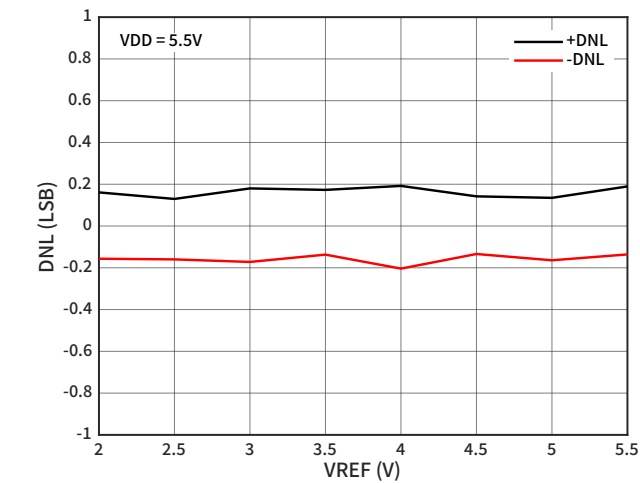
图 8 DNL 误差随 VREF 的变化
