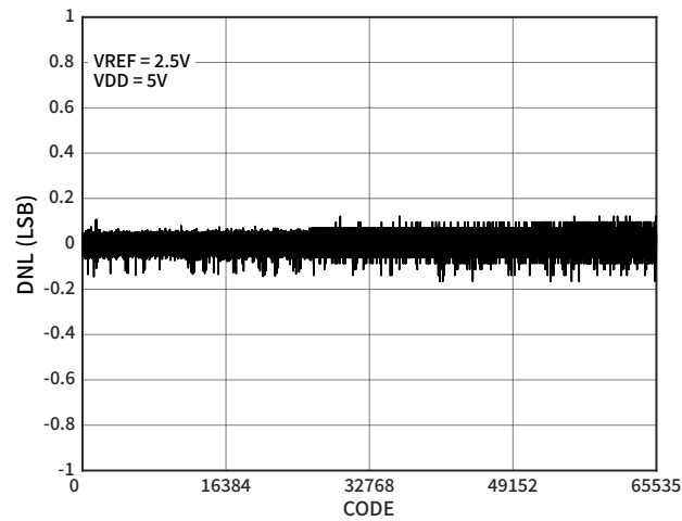
图 6 DNL
