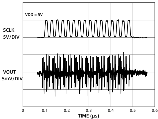
图 19 数字馈通
