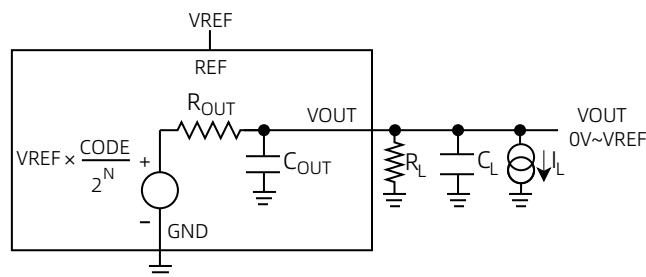
图 24 VOUT 管脚等效电路
