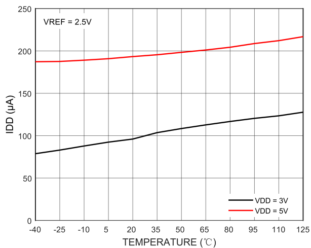
图 16 I_{DD} 的温度特性
