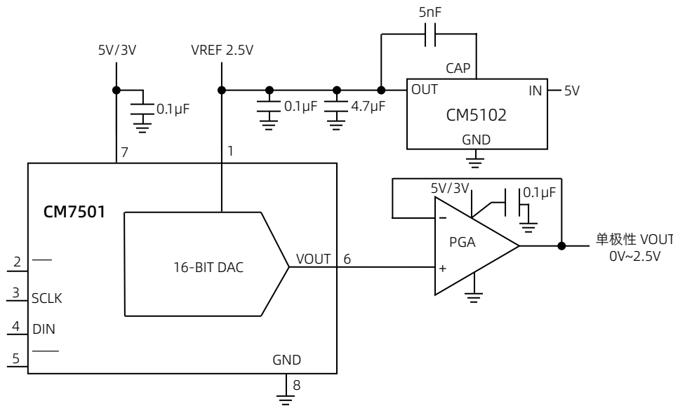
图 26 典型连接
