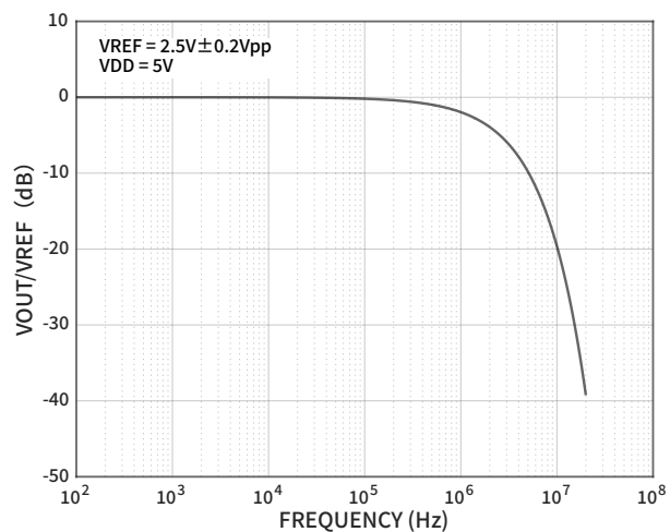
图 18 V_{OUT}/V_{REF}
