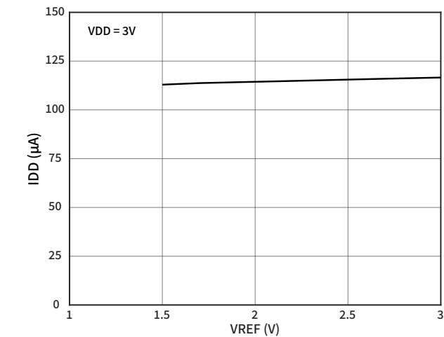
图 12 IDD 随 VREF 的变化 (VDD = 3V)
