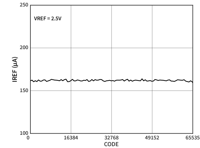
图 10 IREF 随 CODE 的变化
