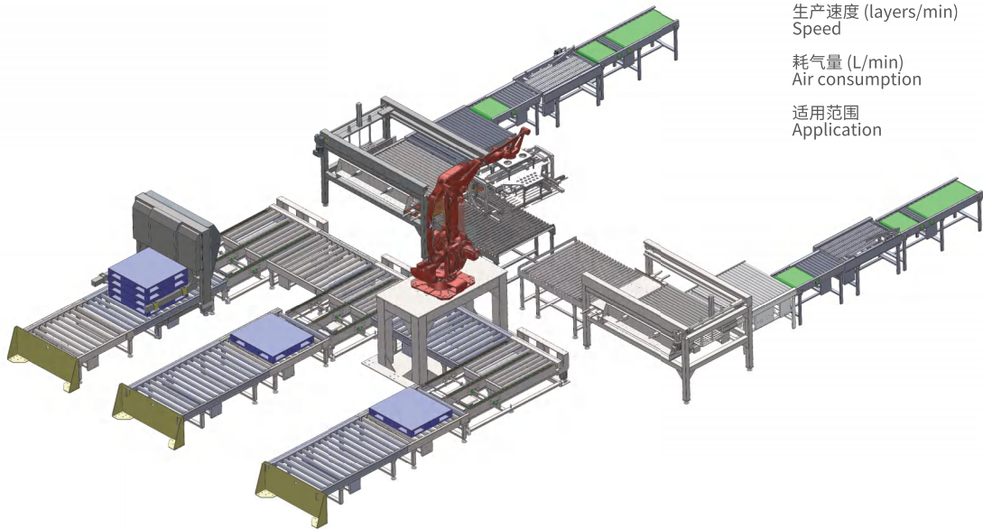
YS-R470-MD45 机器人伺服编组 Robot servo grouping
