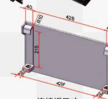
连接板尺寸
