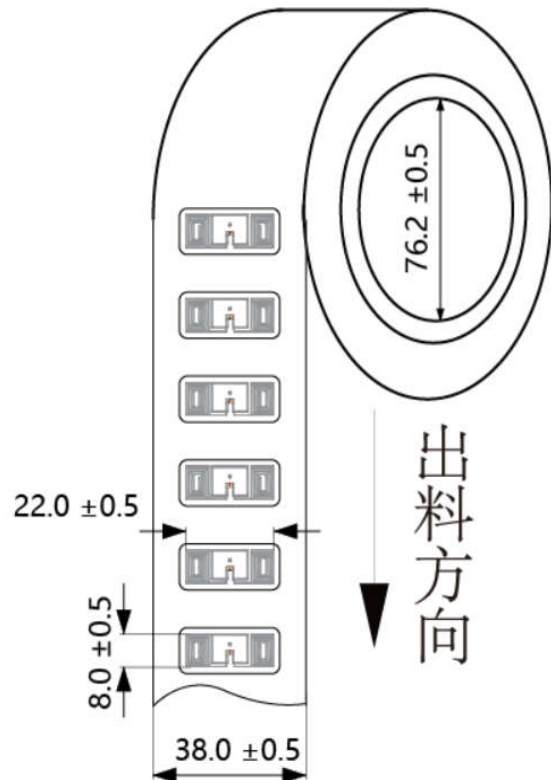
Label 出卷方向示意图
