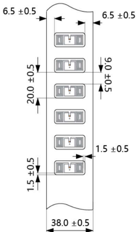
Label 尺寸示意图
