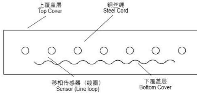
结构示意图
