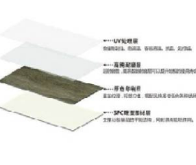
SPC产品结构图
