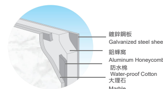
大理石壁板結構 Marble Wall Panel Structure
