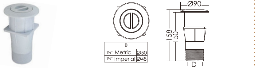
KK-1424
