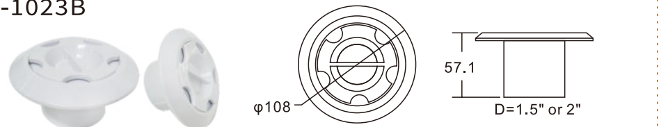
KK-1023B
