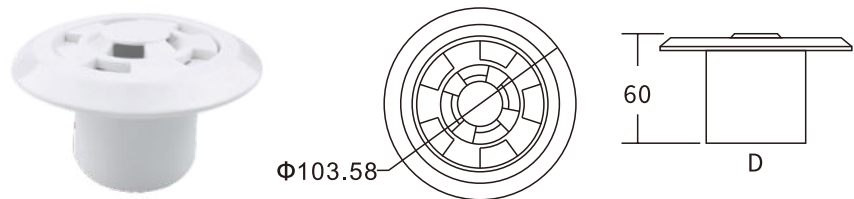
HT-1526W
