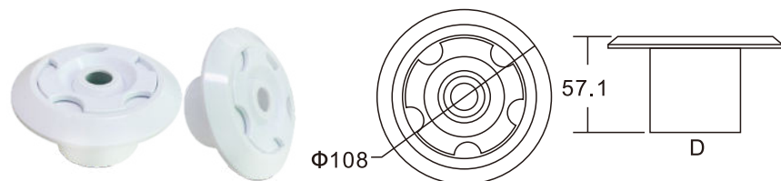
KK-1434
