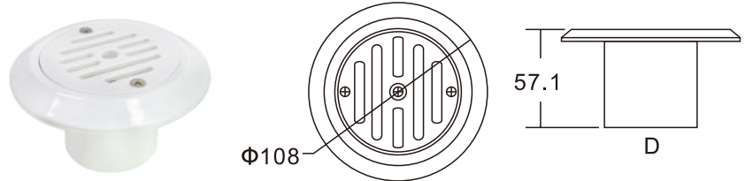
KK-1424B
