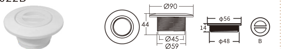
KK-1022B
