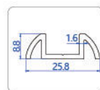
下轨 Bottom track
