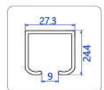
上轨 Top track
