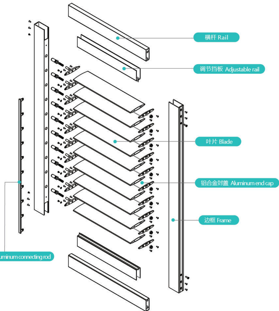
横杆 Rail
