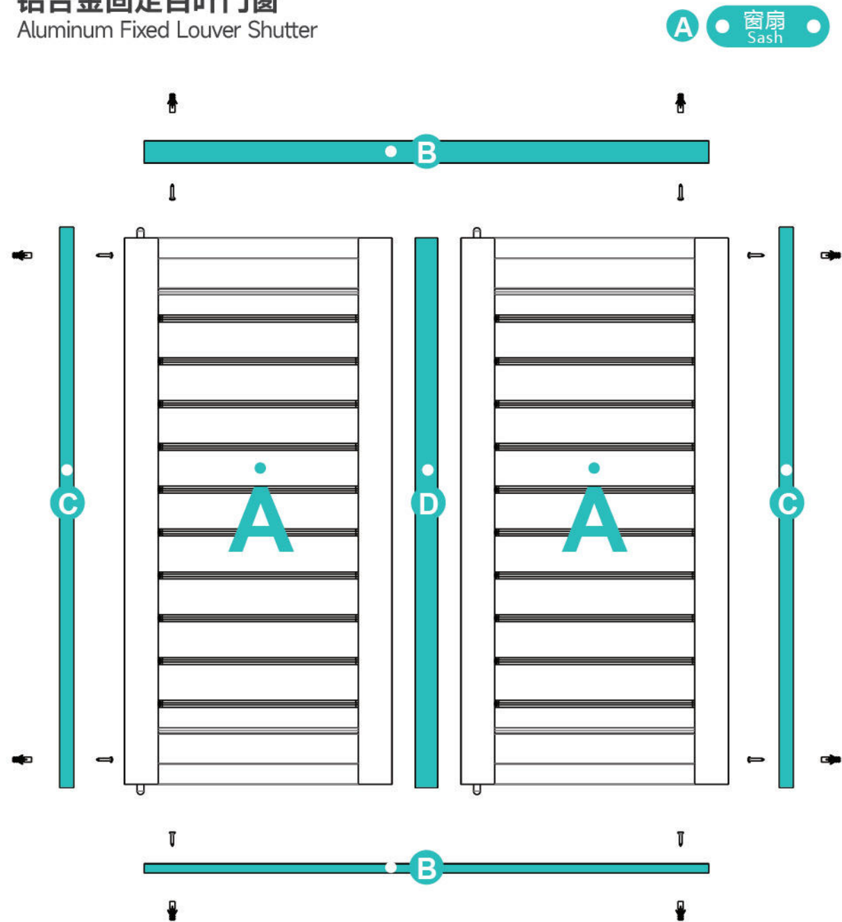
B 上下收边U槽 Top & bottom U channel
