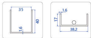
B 上下收边U槽 Top & bottom U channel
