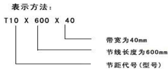
T10 梯形同步带规格、型号、尺寸(节距=10.00mm)
