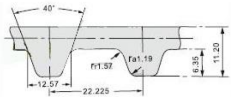
XH齿形图:
