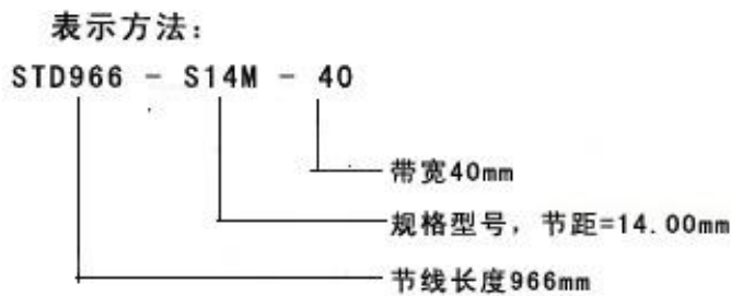
S14M 圆弧齿同步带规格、型号、尺寸(节距=14.00mm)
