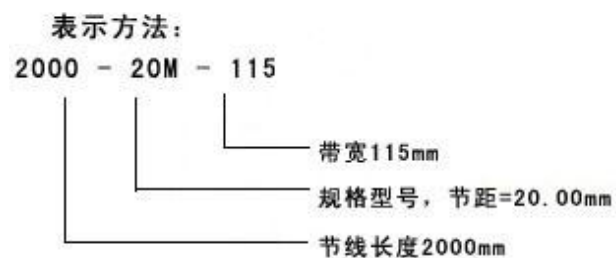
20M 圆弧齿同步带规格、型号、尺寸(节距=20.00mm)
