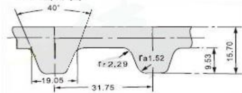
XXH齿形图:
