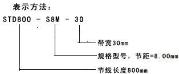
S8M 圆弧齿同步带规格、型号、尺寸(节距=8.00mm)
