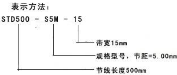
S5M 圆弧齿同步带规格、型号、尺寸(节距=5.00mm)
