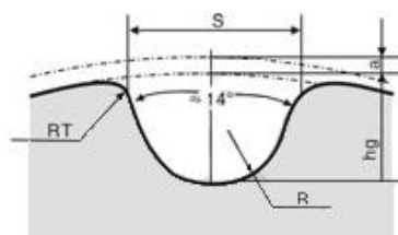
HTD型带轮齿形尺寸
