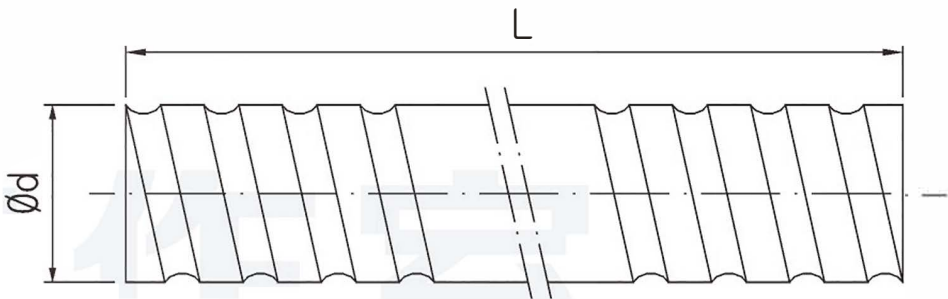
图2.1.1 螺杆示意图
