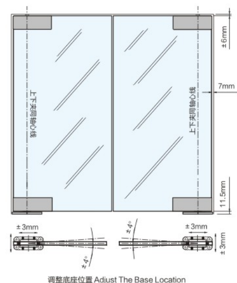
调整底座位置 Adjust The Base Location
