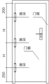
3个液压的安装方法
