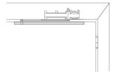
H-2 滑槽外装式 Exterior Chute
