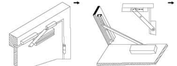
E 滑槽外装式 Exterior Chute
