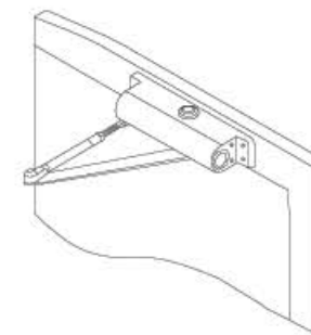
R-2 垂直安装型 (标准型) Regular Arm Application
