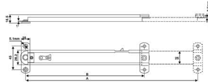
外观尺寸 Dimensions
