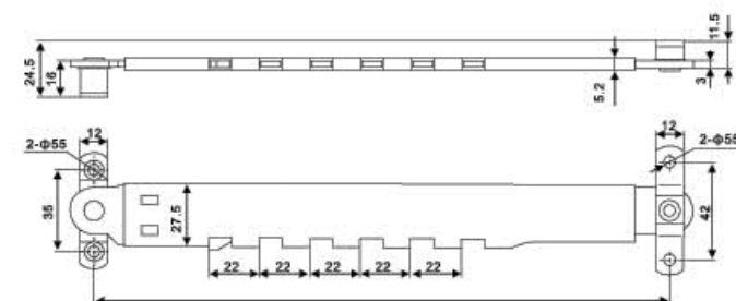
外观尺寸 Dimensions
