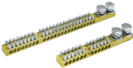
DRB-9x19/24
