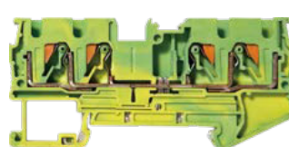
PT 4-QU-PE
