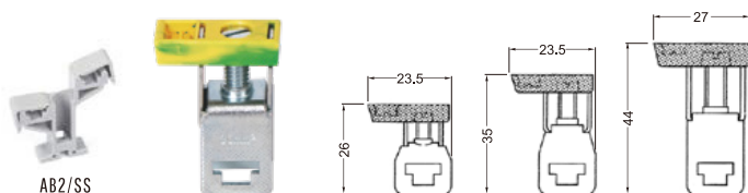
AB2/SS
