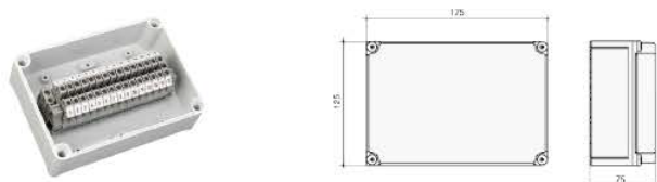
LK171275-10/15P
