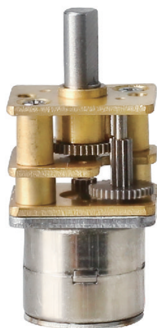
减速箱
