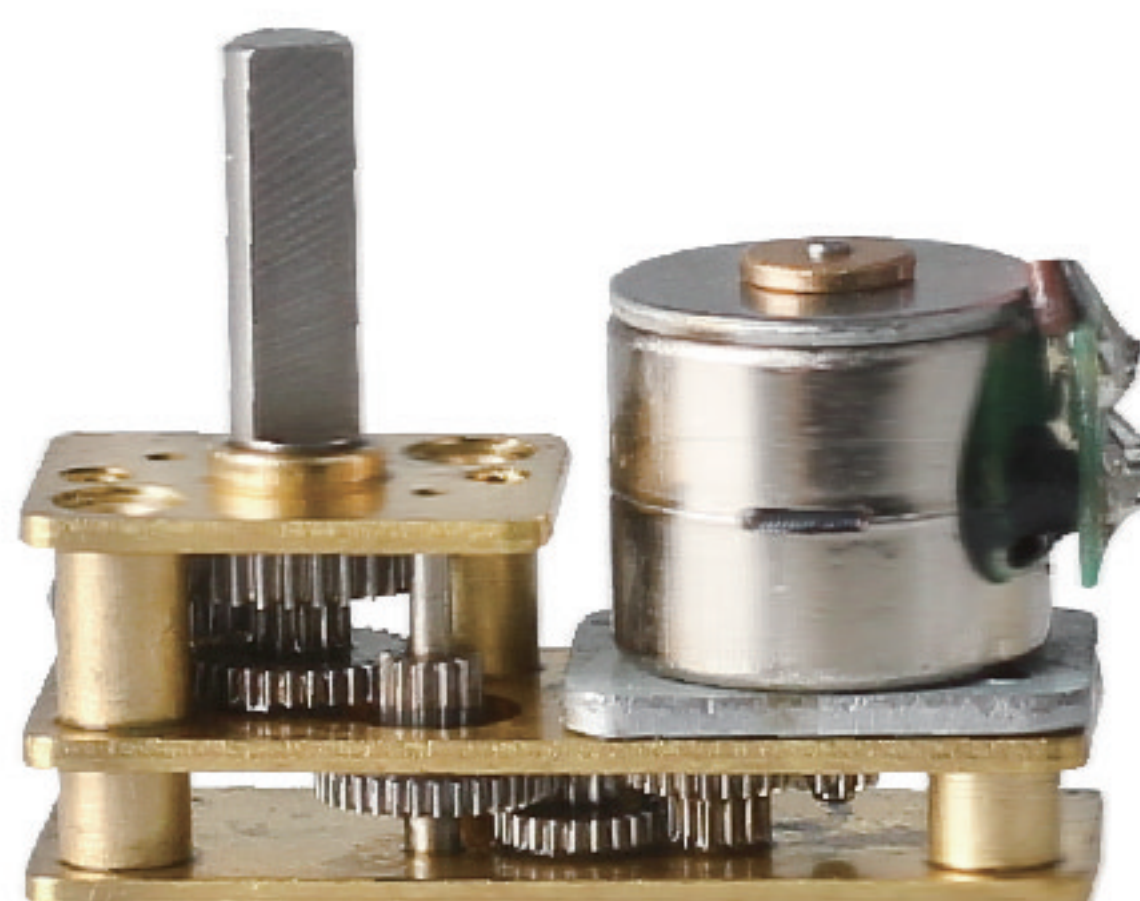
减速箱
