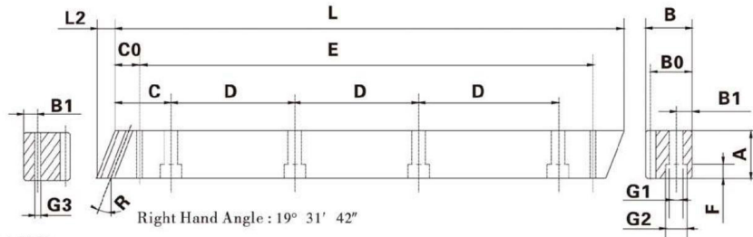
Dimension : mm
