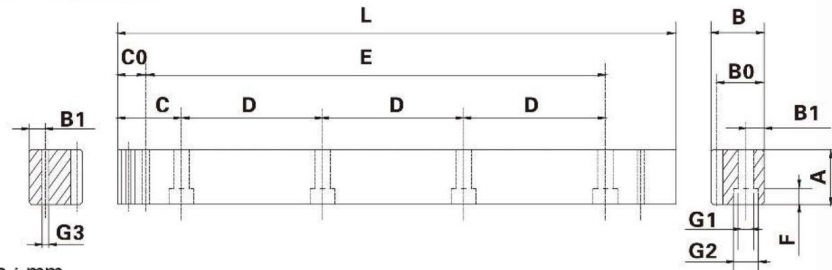
Dimension : mm
