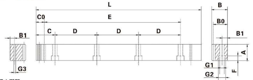
Dimension : mm
