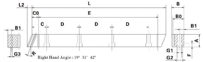
Dimension : mm
