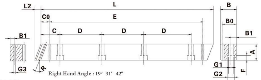
Dimension : mm
