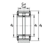
安装尺寸
