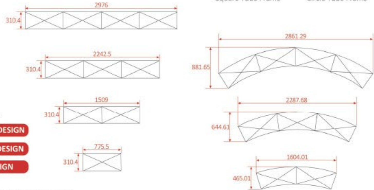
LT-09L2-A Square Tube Frame
