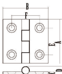
对称合页 Casting Hinge
