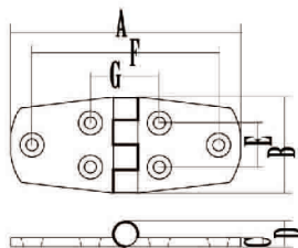
对称合页 Casting Hinge
