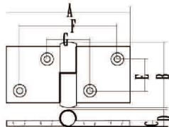
可分离合页 Right Casting Hinge
