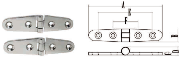
对称合页 Casting Hinge
