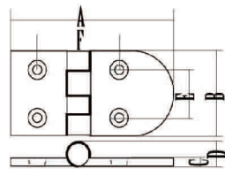
合页 Casting Hinge
