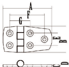
合页 Casting Hinge
