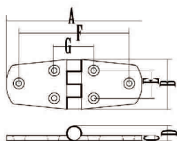
对称合页 Casting Hinge
