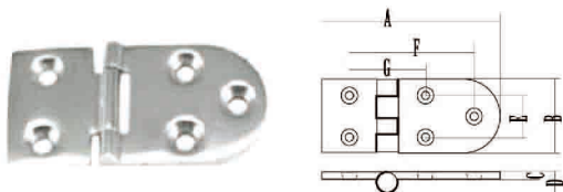
合页 Casting Hinge
