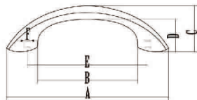
扶手 Lift Handle
